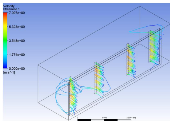
Figura 29 - Simulación a la sala de inversores, donde se aprecia la poca ventilación
