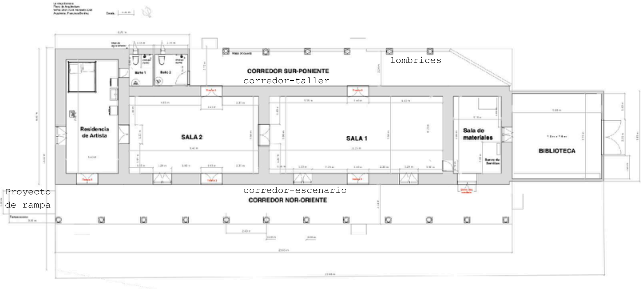
Planta edificio
